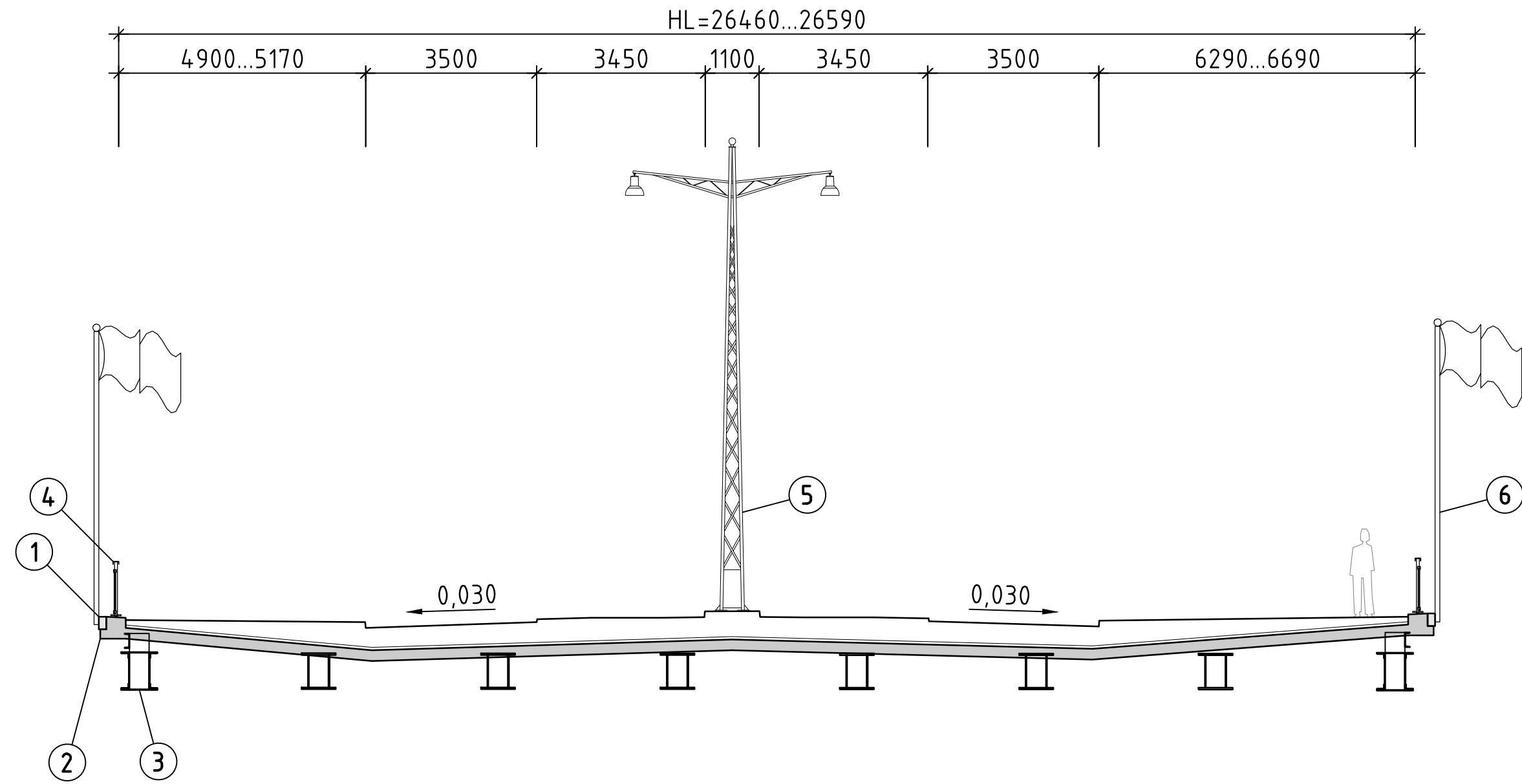
LEIKKAUS B-B, 1:100
