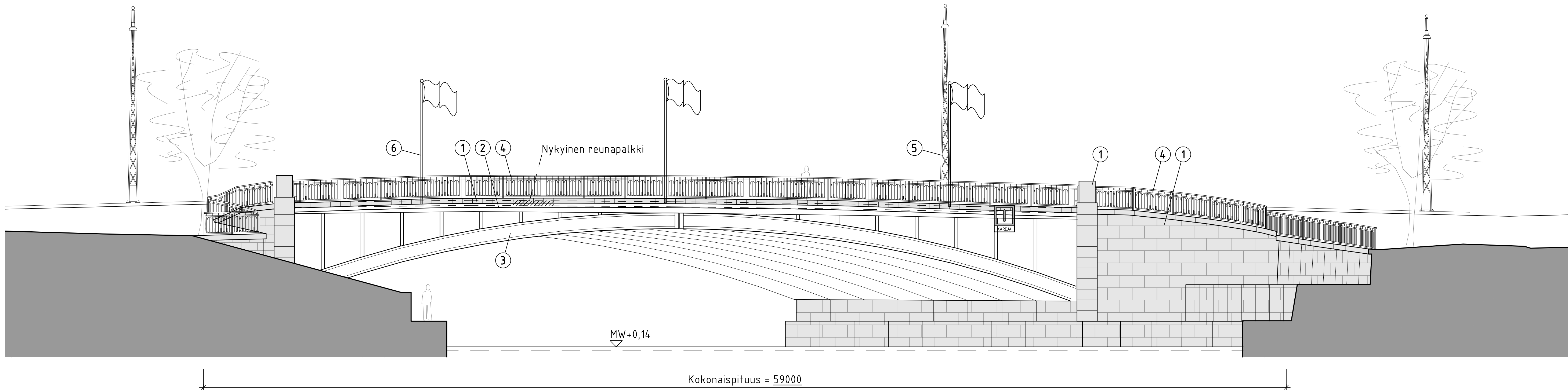
TASO, 1:200
