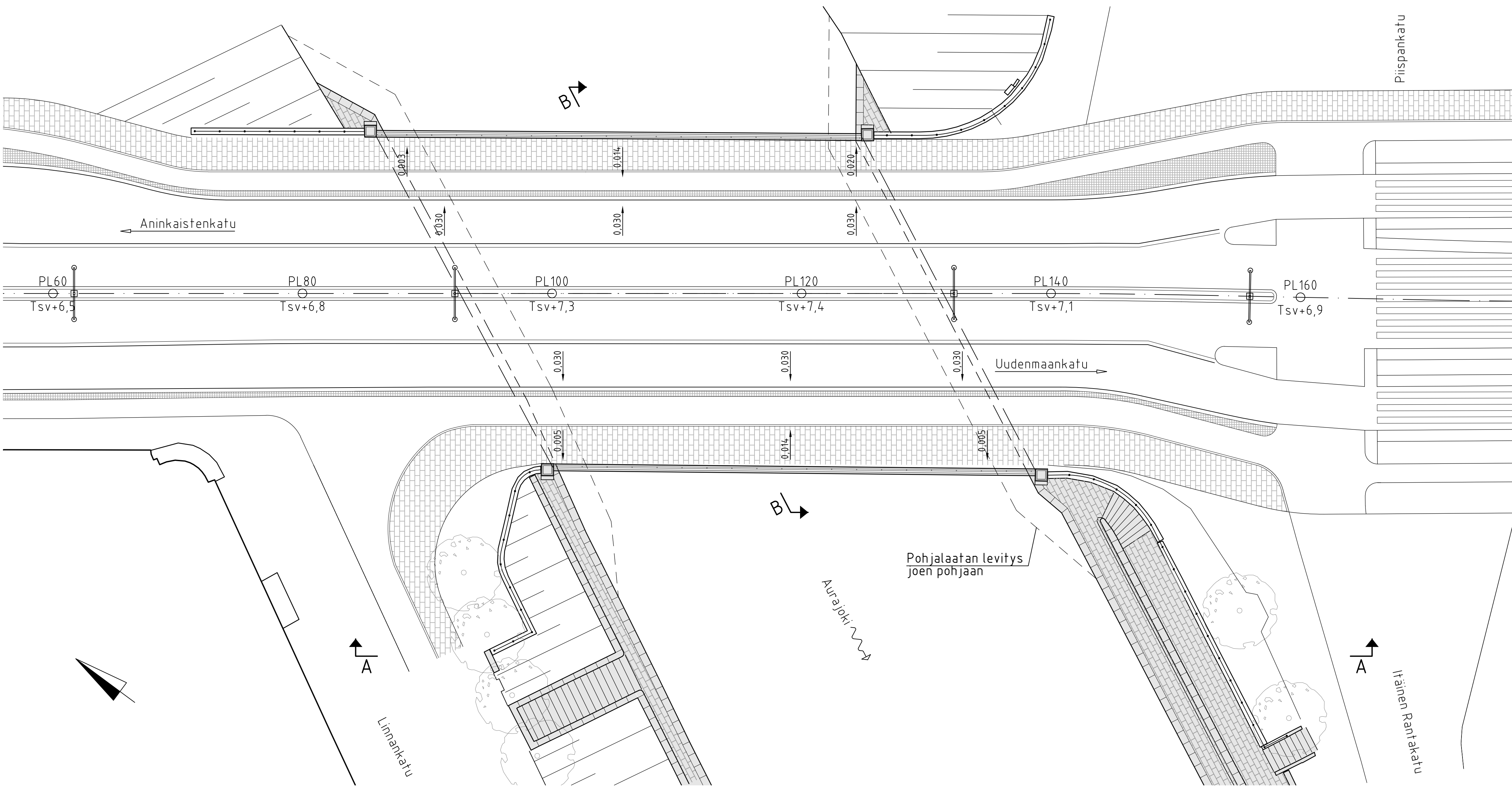
TASO, 1:200
